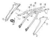
Chasis trasero
